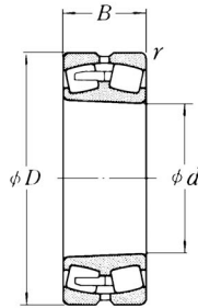
테이퍼구멍
