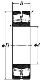
원통구멍
