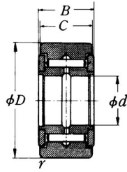
총로울러형
