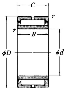
내륜부착 NA
