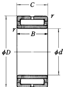
내륜부착 NA
