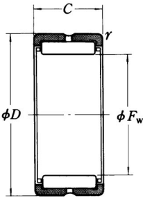
내륜없음 RNA
