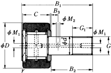
총로울러형
