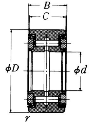
총로울러형
